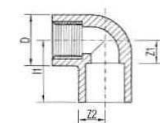
كوع زاوية ٩٠° بسن داخلي
