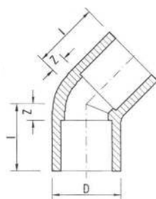
كوع فائق ٤٥°
