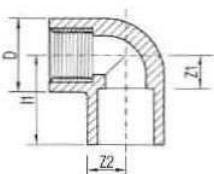
كوع زاوية ٩٠° بسن داخلي
