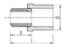
جلبة بسن نحاس خارجي
