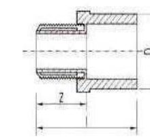
جلبية بسن خارجي
