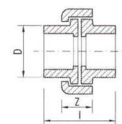
شد وصل
