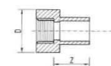
جلبة بسن نحاس داخلي
