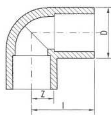
كوع زاوية ٩٠°
