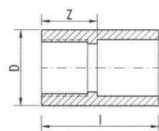
جلبة بسن داخلي
