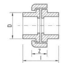
شد وصل
